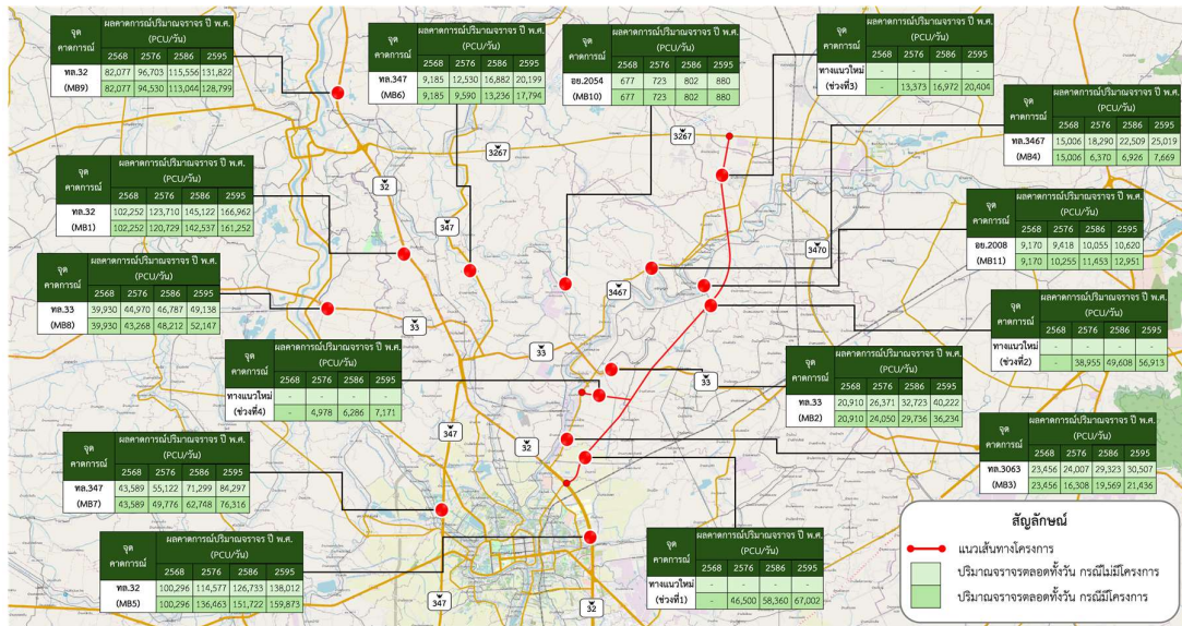
รูปที่ 8.2-2 ผลการคาดการณ์ปริมาณจราจรบนช่วงถนนกรณีมีและไม่มีโครงการ ตลอดทั้งวัน
