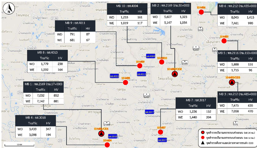
รูปที่ 8.2-1 ผลสำรวจปริมาณจราจรในพื้นที่บริเวณ พท.2169 อ.กุดชุม จ.ยโสธร
