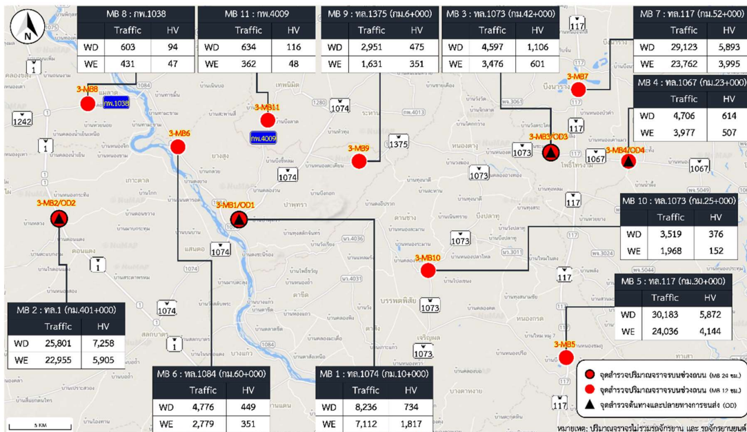
รูปที่ 8.2-1 ผลสำรวจปริมาณจราจรในพื้นที่บริเวณ ทล.1 อ.คลองขลุง จ.กำแพงเพชร
