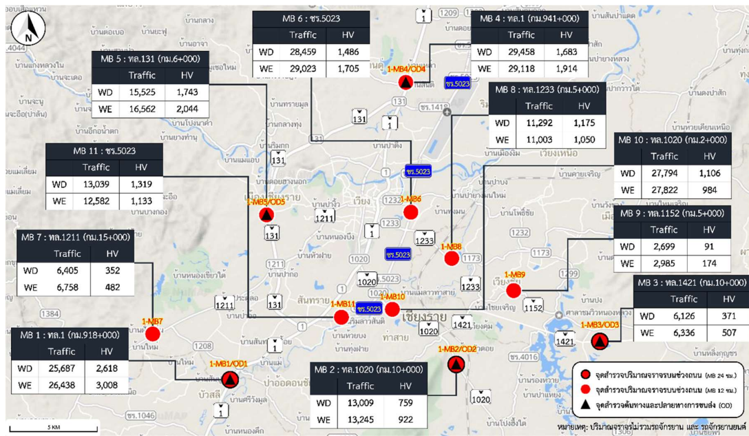
รูปที่ 8.2-1 ผลสำรวจปริมาณจราจรในพื้นที่บริเวณ พท.1020 อ.เมืองเชียงราย จ.เชียงราย
